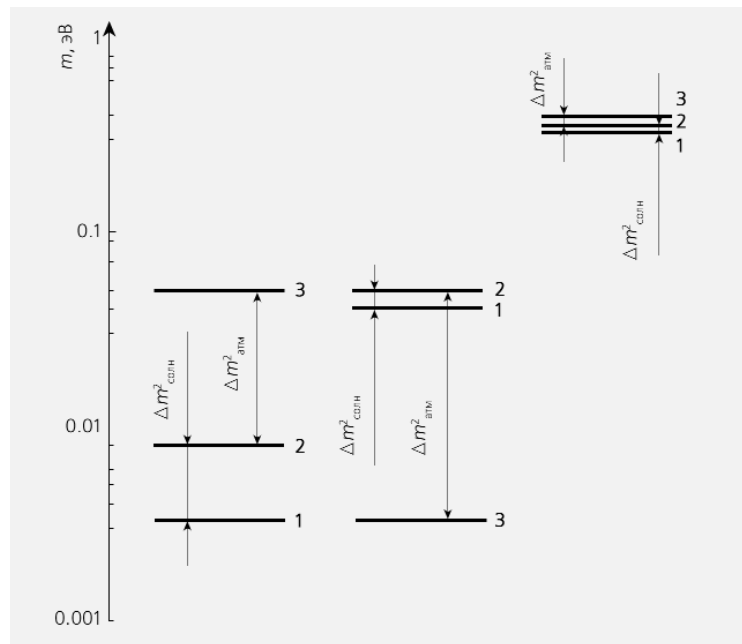
Рис.1. Прямая, инвертированная и вырожденная схемы масс нейтрино.
