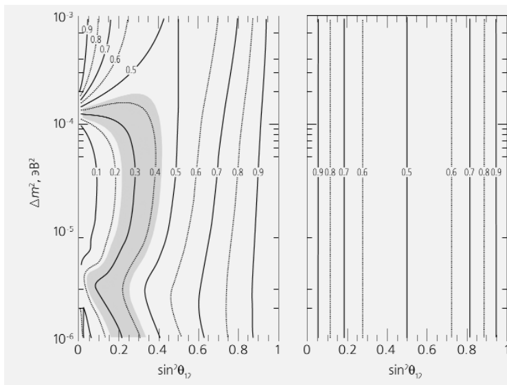
Рис.2. Изолинии вероятности выживания электронных нейтрино от распада 8 B. Слева — когда работает МСВ-эффект, справа — для чисто вакуумных осцилляций.
