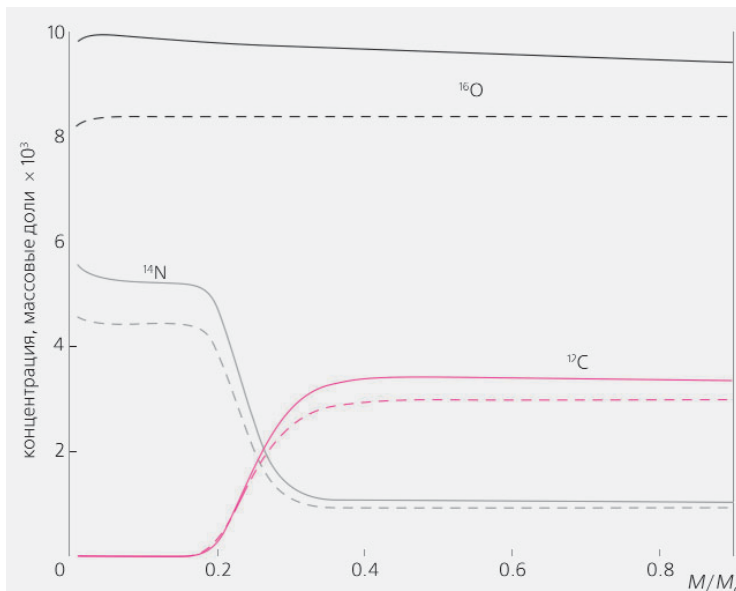
Рис.4. Распределение концентраций ^{12}\text{C} , ^{14}\text{N} и ^{16}\text{O} по радиусу Солнца. Сплошные линии — данные расчета с учетом диффузии элементов в веществе Солнца, штриховые — без ее учета.
