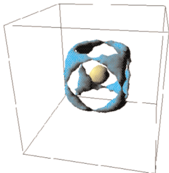
Рис.5. Пространственное распределение плотности атомов дейтерия в элементарной ячейке \text{ND}_4\text{Cl} , усредненное во времени.
