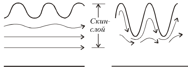
Рис.8. Скин-эффект на шероховатой поверхности
