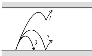
Рис.4. Движение электронов в ЭВП со скрещенными полями при взаимодействии с электромагнитной волной
