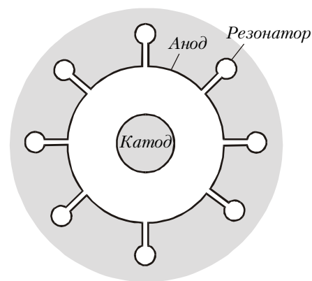
Рис.5. Магнетрон с резонаторами типа «цель-отверстие»
