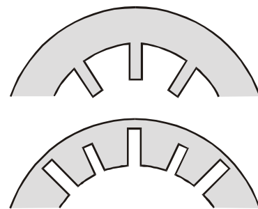
Рис.6. Замедляющие системы магнетронов: вверху – лопаточного типа, внизу – щелевого типа
